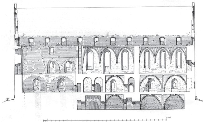
15. Działdowo, przekrój przez główne skrzydło zamku: na piętrze kaplica i refektarz. Repr. wg Conrad Steinbrecht, Die Ordensburgen der Hochmeisterzeit , Berlin 1920, il. 119
