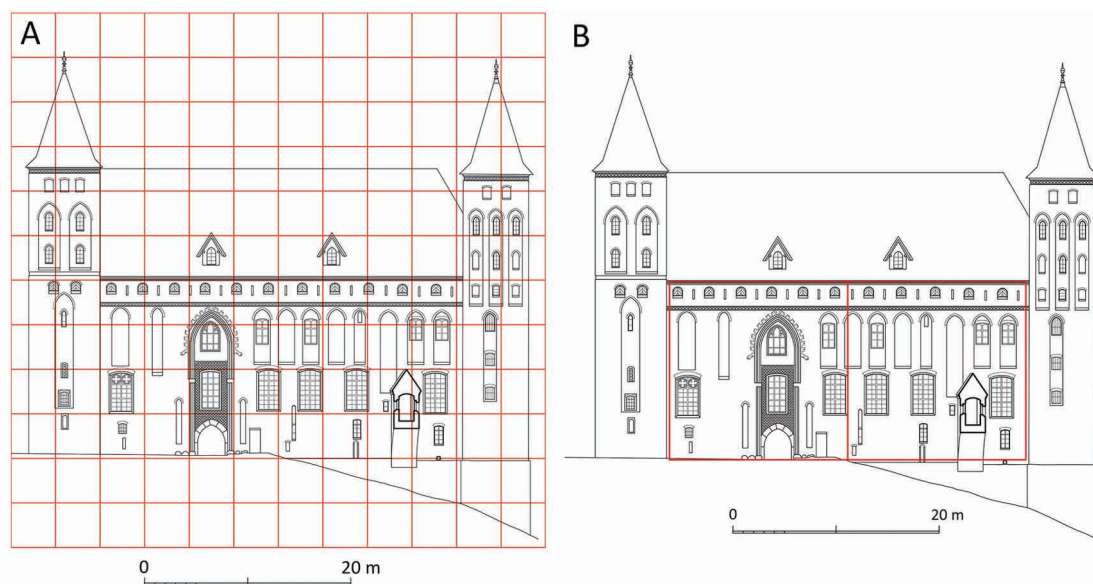
8. Kwidzyn, północna elewacja kasztelu (stan po przebudowach z XIX–XX w.): A – na siatce o module 1 pręta nowej miary chełmińskiej; B – proporcje elewacji. Oprac. Bogusz Wasik według inwentaryzacji Ireny Jaroszewskiej-Bartoszewicz
