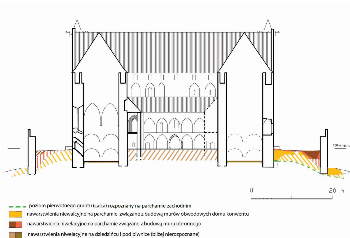
14. Radzyń Chełmiński, przekrój przez dom konwentu. Przykład zakresu prac ziemnych (nasypowych) w tzw. klasycznym zamku konwentualnym. Oprac. Bogusz Wasik
