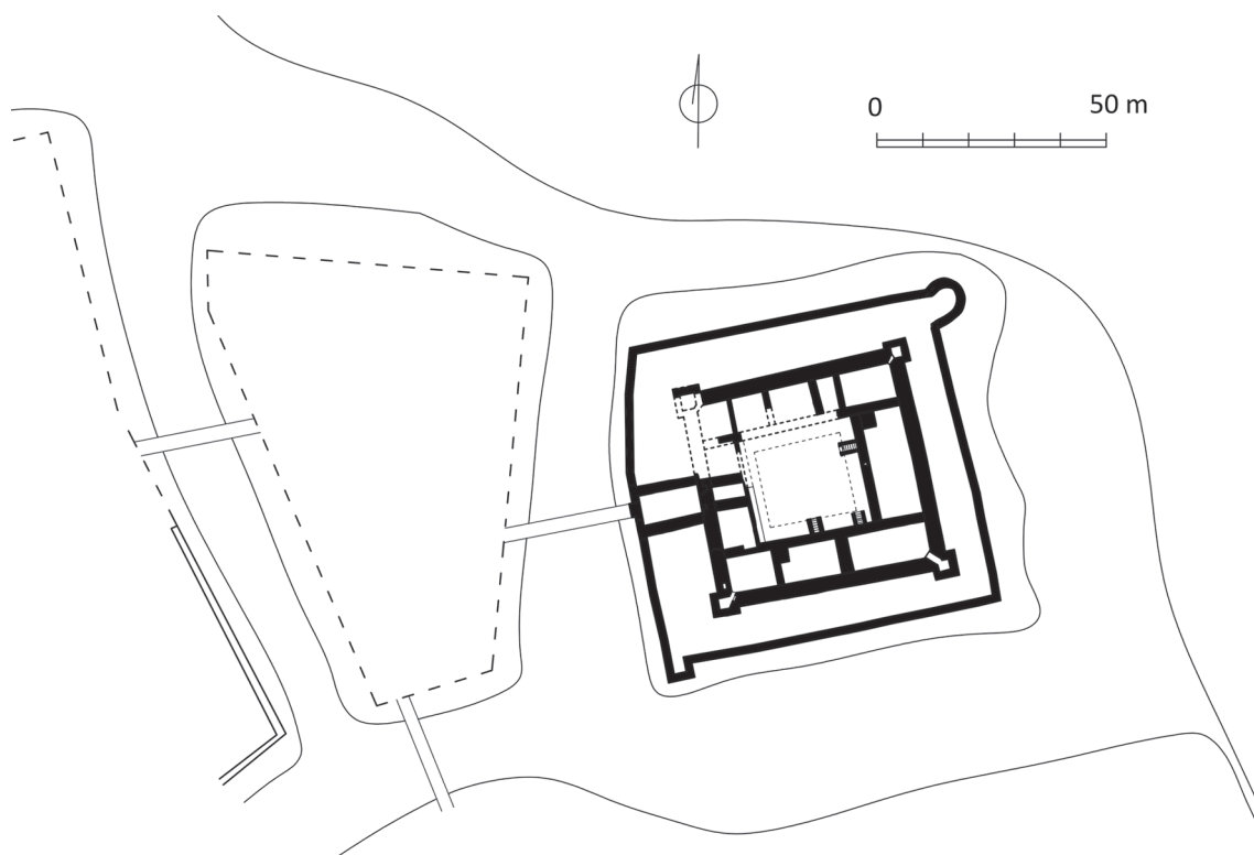
3. Lubawa, rzut zamku według badań z lat 1998–2001 i 2015–2016. Rys. Bogusz Wasik
