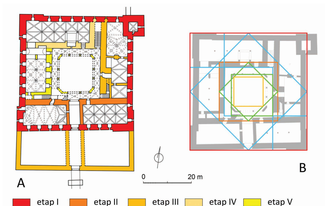
11. Lidzbark Warmiński, zamek wysoki (kasztel): A – rzut etapów budowy I fazy z ok. 1350–1373 r. Rys. Bogusz Wasik według badań Wojciecha Wólkowskiego; B – rzut I fazy zamku z wyznaczeniem proporcji metodą ad quadratum . Oprac. Bogusz Wasik
