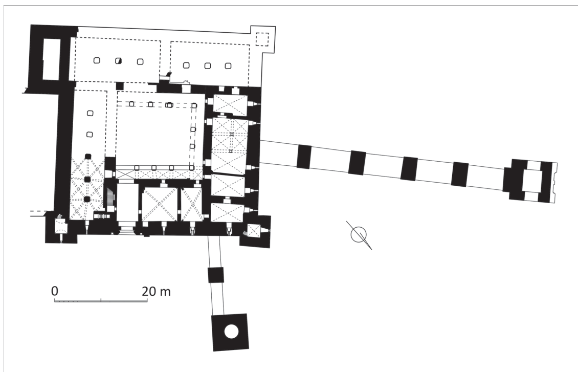
7. Lubawa, rekonstrukcja średniowiecznego rzutu parteru kaszteleu. Rys. Bogusz Wasik według badań Anny Chrzanowicz
