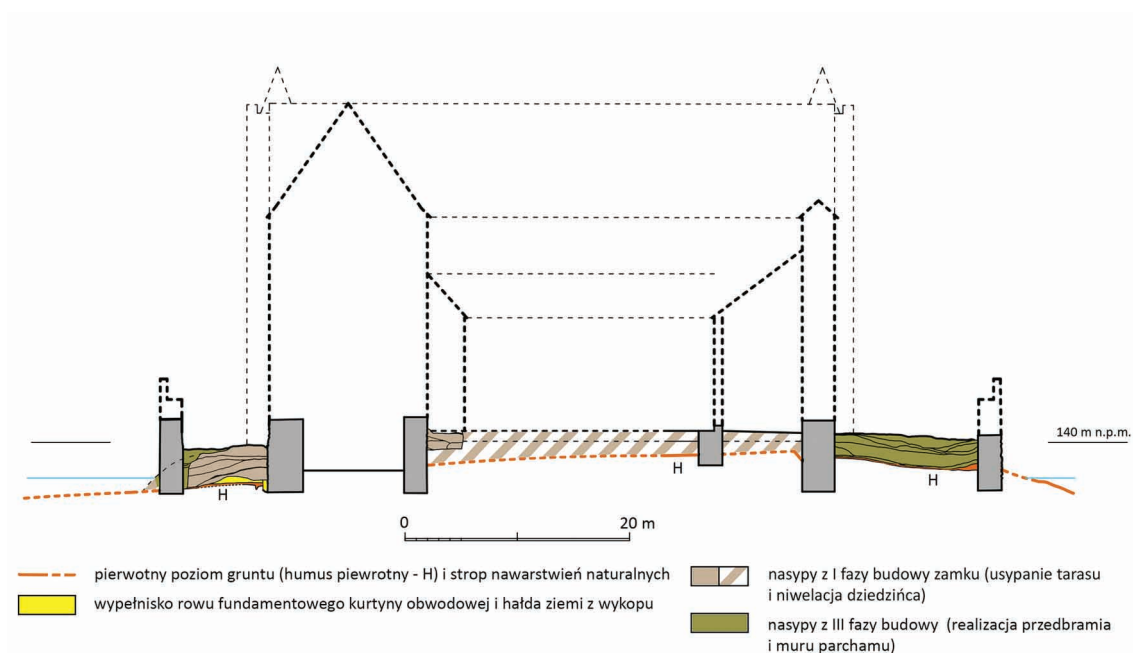
6. Lubawa, przekrój zachód-wschód (widok na południe) zamku wysokiego z zaznaczeniem poziomu gruntu sprzed budowy i nasypów z I i III fazy według badań Leszka Kajzera i Adama Mackiewicza z lat 1998–2001 i 2015–2016. Rys. Bogusz Wasik
