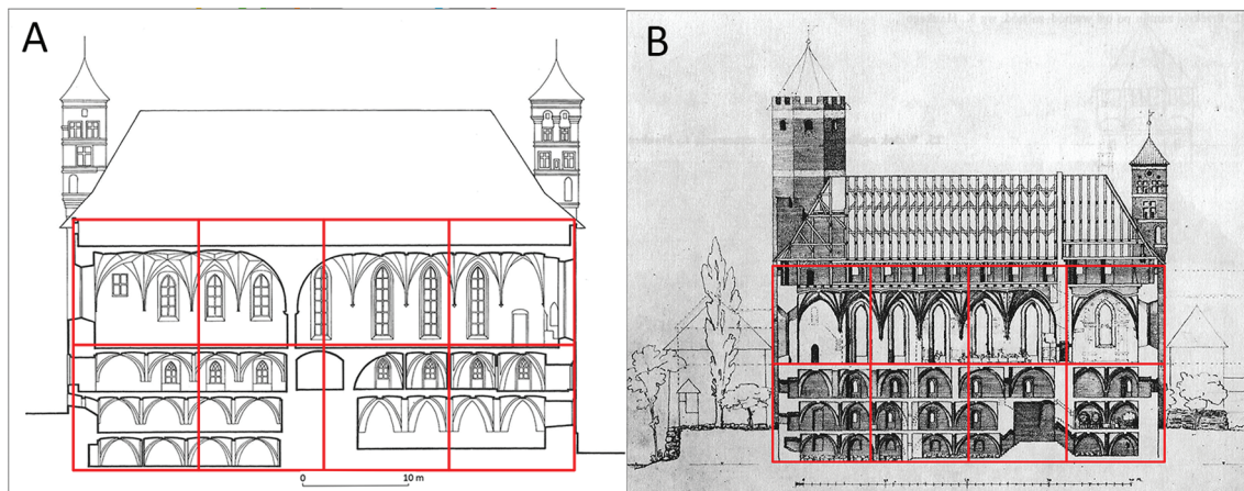
12. Lidzbark Warmiński, przekroje skrzydeł zamku wysokiego (kasztelu) z zaznaczeniem proporcji przy pomocy kwadratów:
