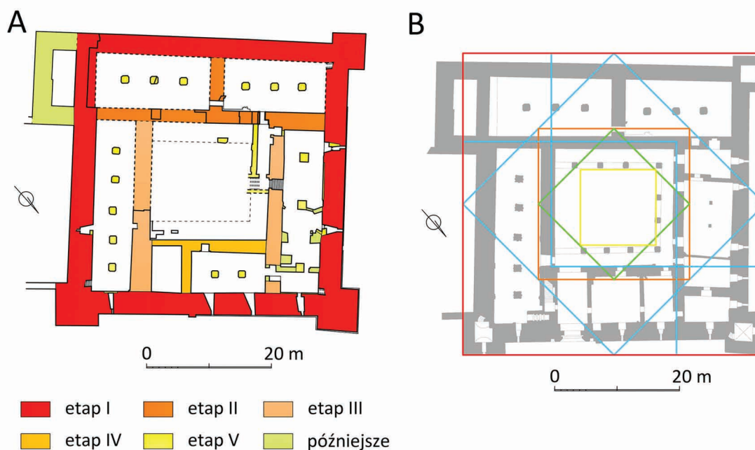
9. Kwidzyn, rzut zamku wysokiego (kasztełu): A – etapy budowy; B – rozrys ad quadratum. Rys. Bogusz Wasik
