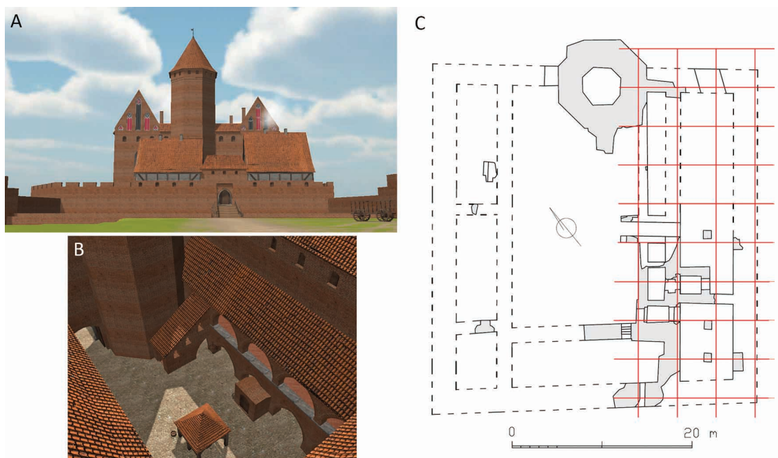
2. Wąbrzeźno, zamek wysoki: A – widok od przedzamcza (stan z początku XVII w.); B – rekonstrukcja dziedzińca z murowanymi schodami prowadzącymi na ganek skrzydła głównego. Koncepcja Bogusz Wasik, wizualizacja Paweł Moszczyński; C – rzut kaszteleu z siatką o module 1 pręta nowej miary chełmińskiej na skrzydle głównym i ganku. Rys. Bogusz Wasik
