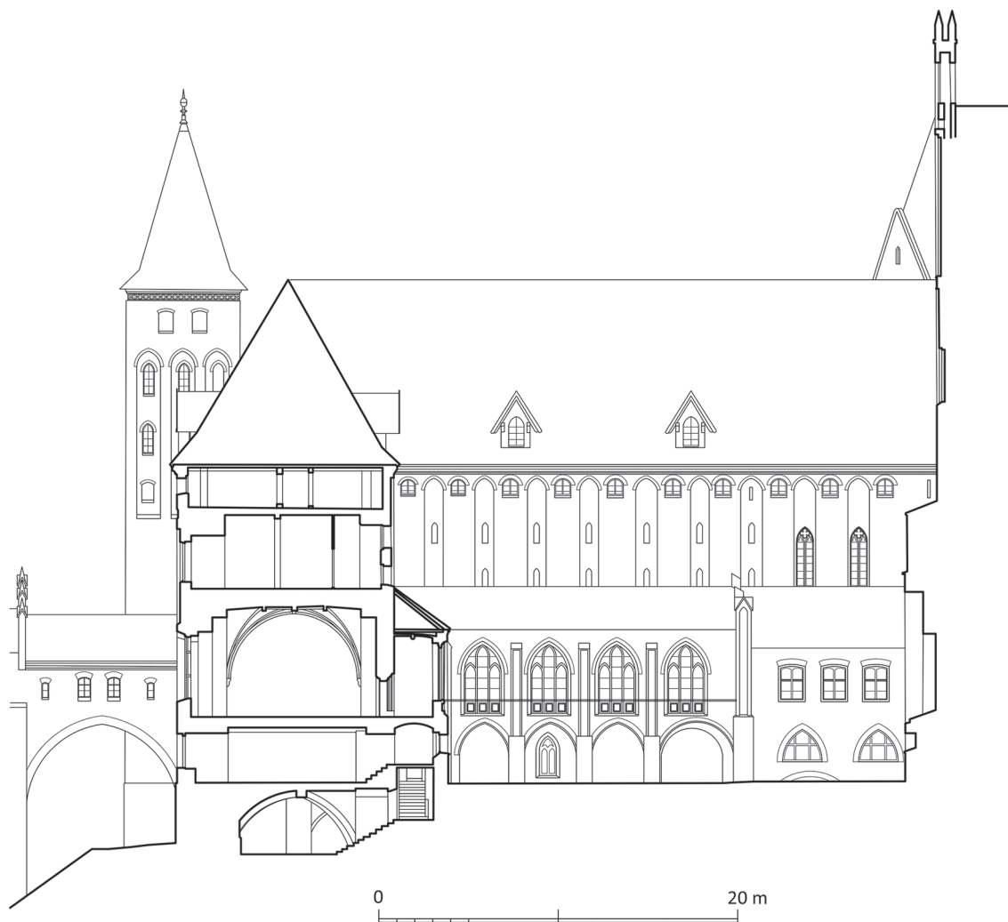
10. Kwidzyn, przekrój zachód-wschód (widok na północ) przez kasztel (stan po przebudowach z XIX–XX w. Rys. Bogusz Wasik według inwentaryzacji Ireny Jaroszewskiej-Bartoszewicz
