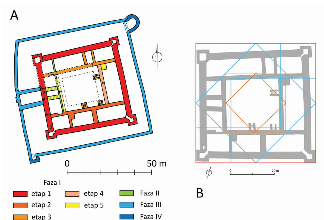
5. Lubawa, rzut zamku wysokiego (kasztelu): A – fazy i etapy budowy; B – rozrys ad quadratum. Rys. Bogusz Wasik
