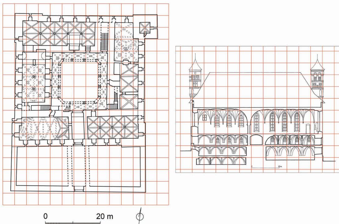
13. Lidzbark Warmiński, zamek wysoki (kasztel) na siatce o module 1 pręta nowej miary chełmińskiej: A – rzut I fazy zamku; B – przekrój skrzydła głównego (południowego) po przebudowach z XV–XVI w. Oprac. Bogusz Wasik według Wojciecha Wólkowskiego (rzut) i Architektura gotycka w Polsce, Warszawa 1995, t. 2, s. 447 (przekrój)
